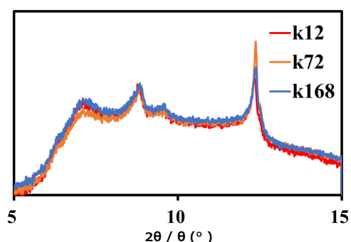
図 2 固液接触時間が異なる黒ボク土試料における X 線回析図
