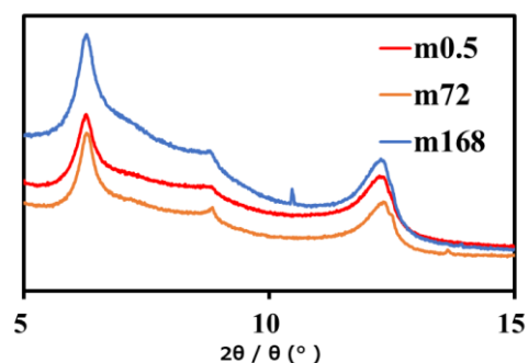
図 1 固液接触時間が異なる真砂土試料における X 線回析図
